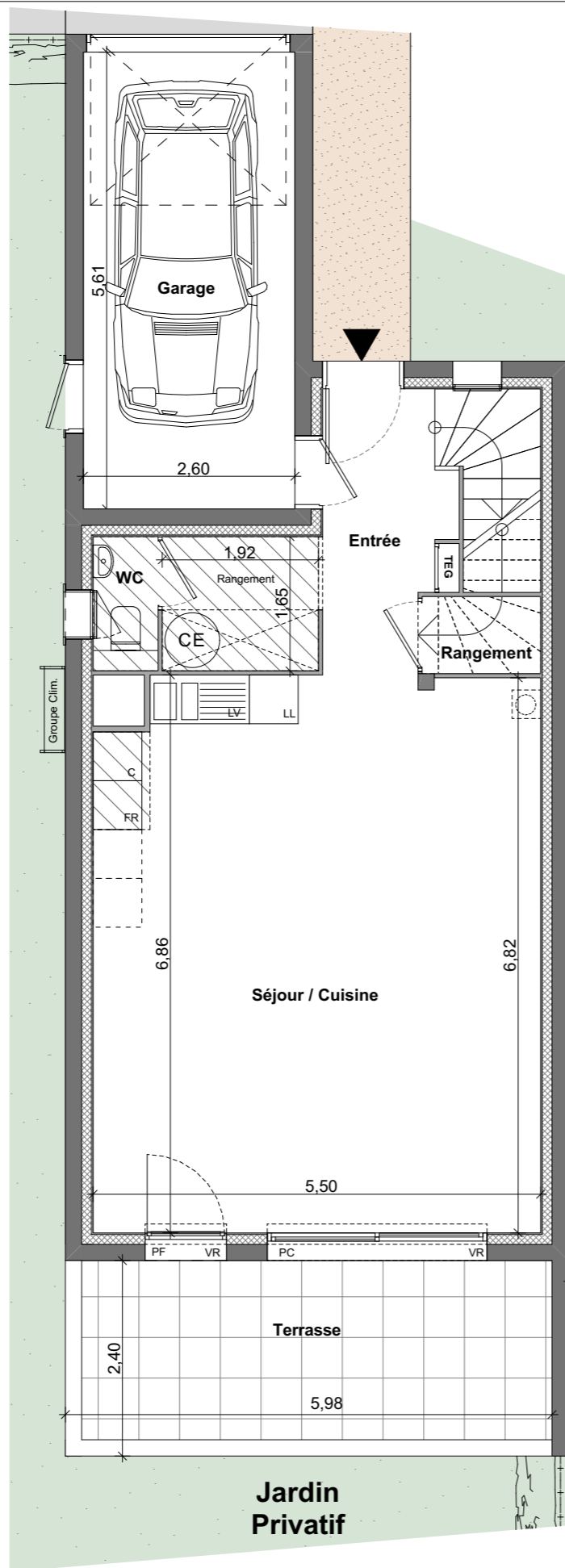
Plan Rez de Chaussée - 1:75
